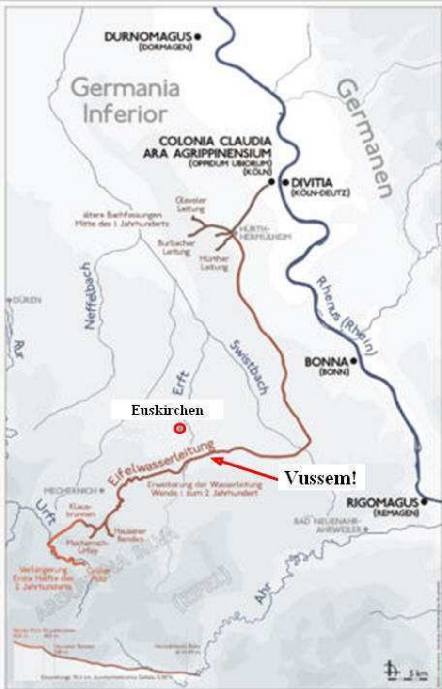
Verlauf der Eifelwasserleitung
